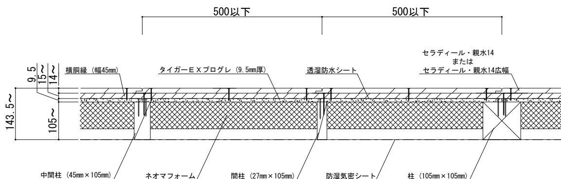
【サイディング縦張り（横胴縁）仕様】
