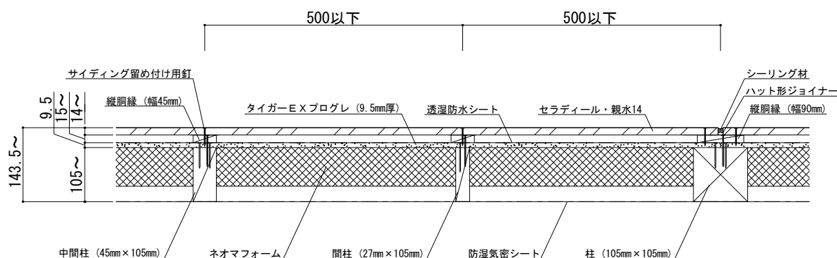
【サイディング横張り（縦胴縁）仕様】
